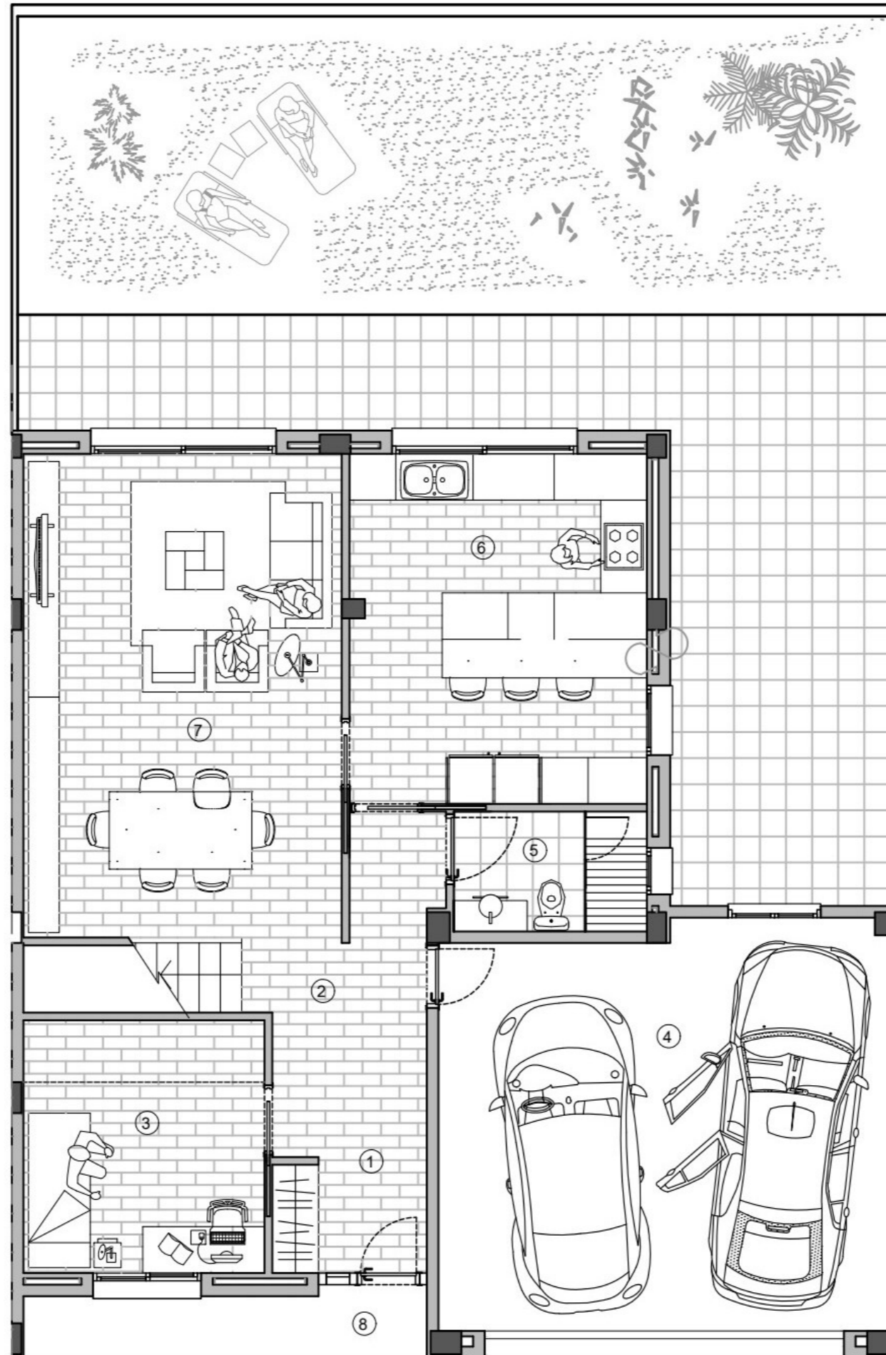
PLANTA BAIXA
